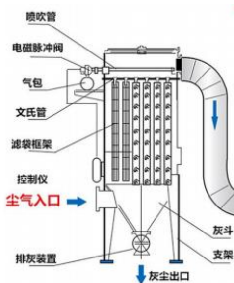
图 4.1.2-1 袋式除尘器工作原理图
